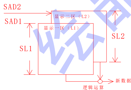
(a) 单屏结构：显示一，二区参加的二重合成显示方式
